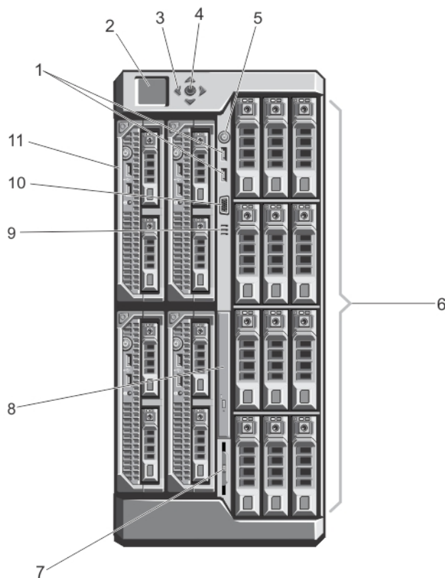
图 3: 前面板功能部件和指示灯 - 3.5 英寸硬盘驱动器机箱
